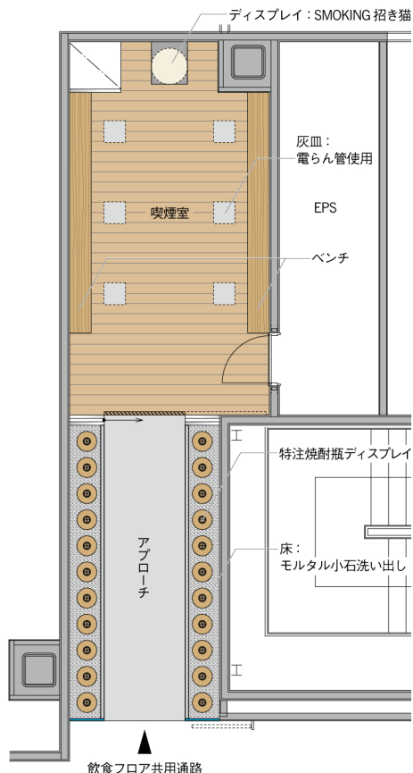
屋内喫煙スペース PLAN 1：100
